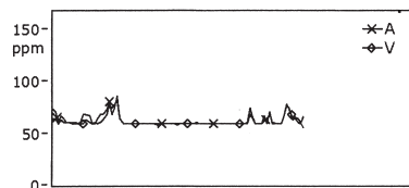
Abb. 5a: DDD 60/Min (keine Frequenzanpassung, Daten der Austrittskontrolle)
