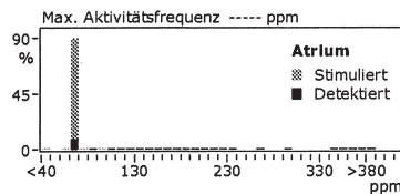
Abb. 5a: DDD 60/Min (keine Frequenzanpassung, Daten der Austrittskontrolle)
